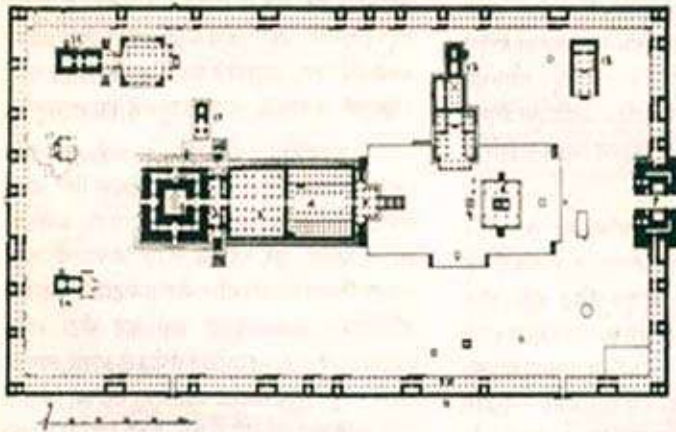
आकृति १ - बृहदीश्वर प्रासादाचा अपोच्छंद
